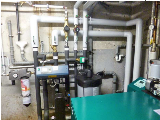
Wärmetauscher für Warmwasser für die Zapfstellen;
